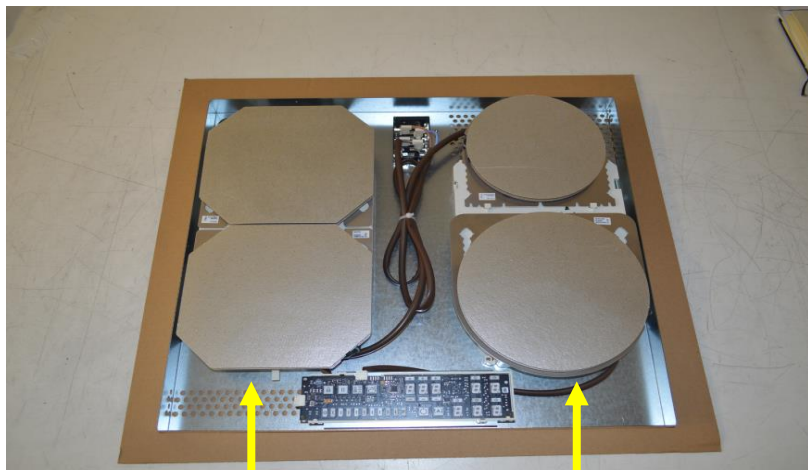
Master Module
