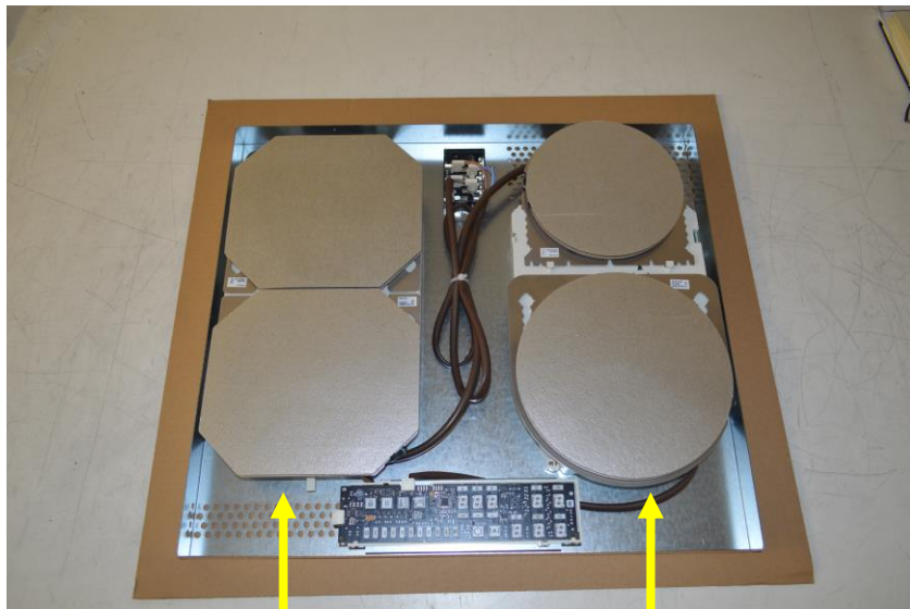
Master Module
